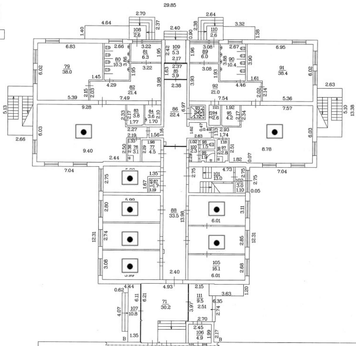
Būves daļējuma shēma
